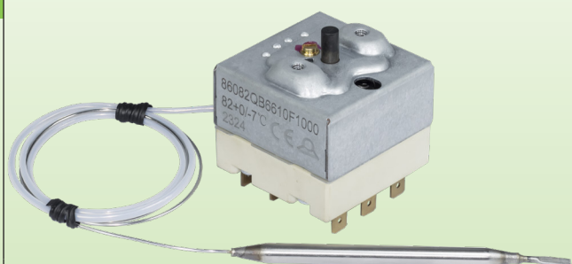
Тип с креплением при помощи центральной втулки М10
